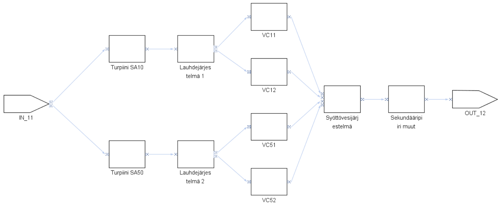
Kuva L1-3. Yleismallin käytettävyyslohkokaaviot Miriam RAM Studiossa - sekundääripiirin sisäinen rakenne.
