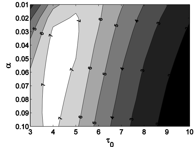
Kuva 1 Option arvo arviointivirheen keskihajonnan \tau_0 ja kynnsarvon \alpha funktiona
