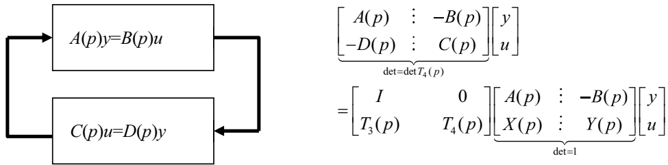
Kuva 1. Monimuuttujasäätö
